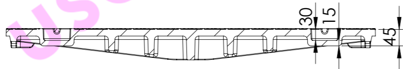
COUPE A-A
